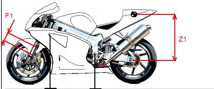
Angehobenes Motorrad
