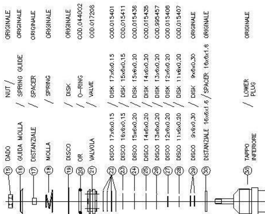
SCHEMA 'B' GRUPPO COMPRESSIONE SCHEME 'B' COMPRESSION SET
